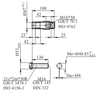
GFV/GFVZ/GFVF67输出轴
