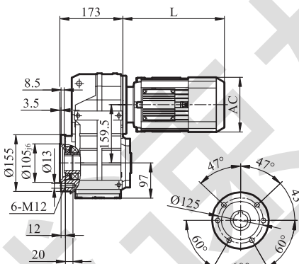
GFAZ/GFHZ/GFVZ67
