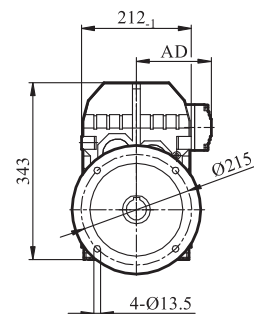
GFV/GFVZ/GFVF67输出轴
