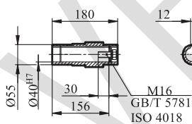
GFA/GFAZ/GFAF67输出轴
