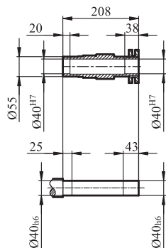
GFH/GFHZ/GFHF67输出轴
